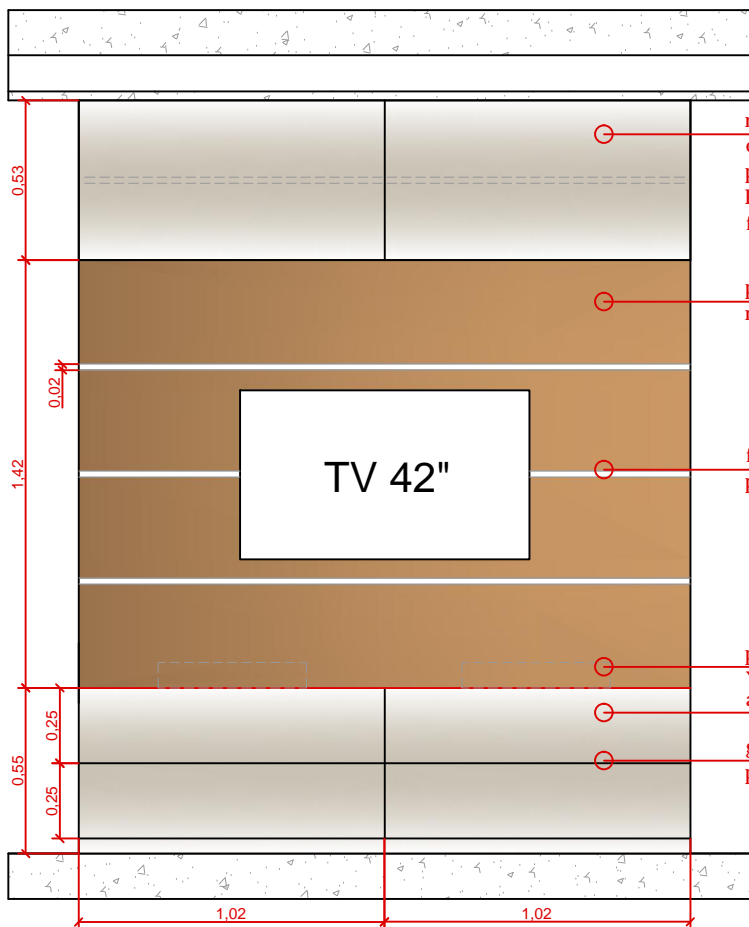
móvel tv vista esc: 1.25
